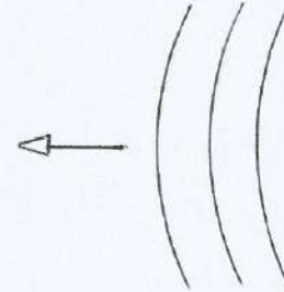
Frente de onda V = 300.000 \text{ km/s}
